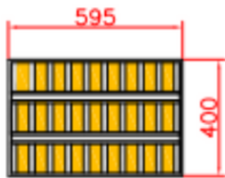
DIMENSÕES DA BANDEJA
